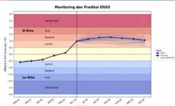
Grafik B1.1. Monitoring dan Prediksi ENSO
