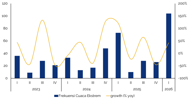
Grafik 2.6. Frekuensi Cuaca Ekstrem
